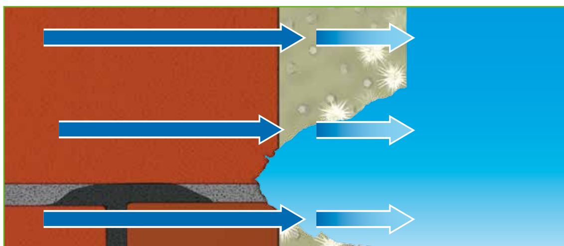
Tuhoisa kristalloitumisprosessi
